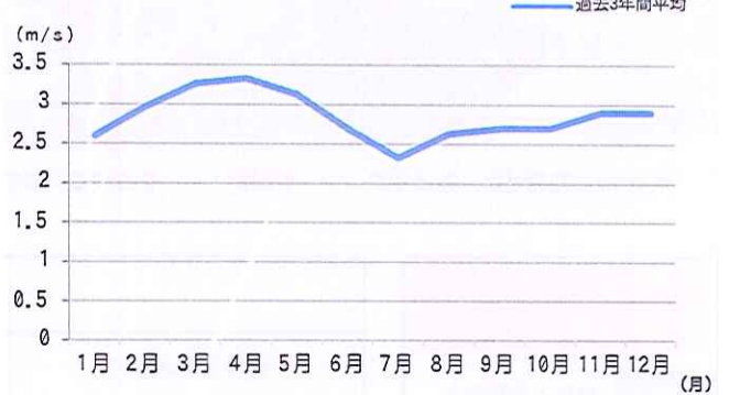
月平均風速
