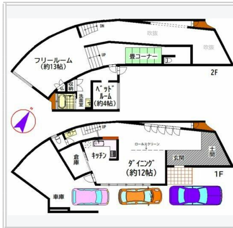
間取り図
