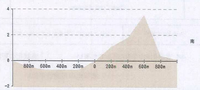
南北高低差 (m)
