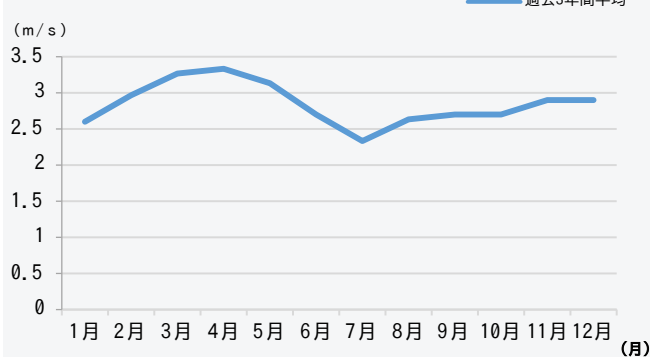
月平均風速
